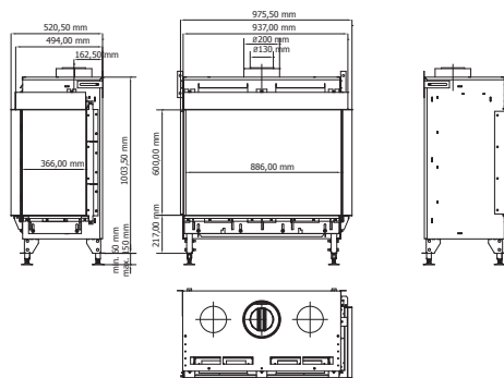
Monroe - FR 900
