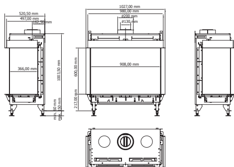
Monroe - LFR 900
