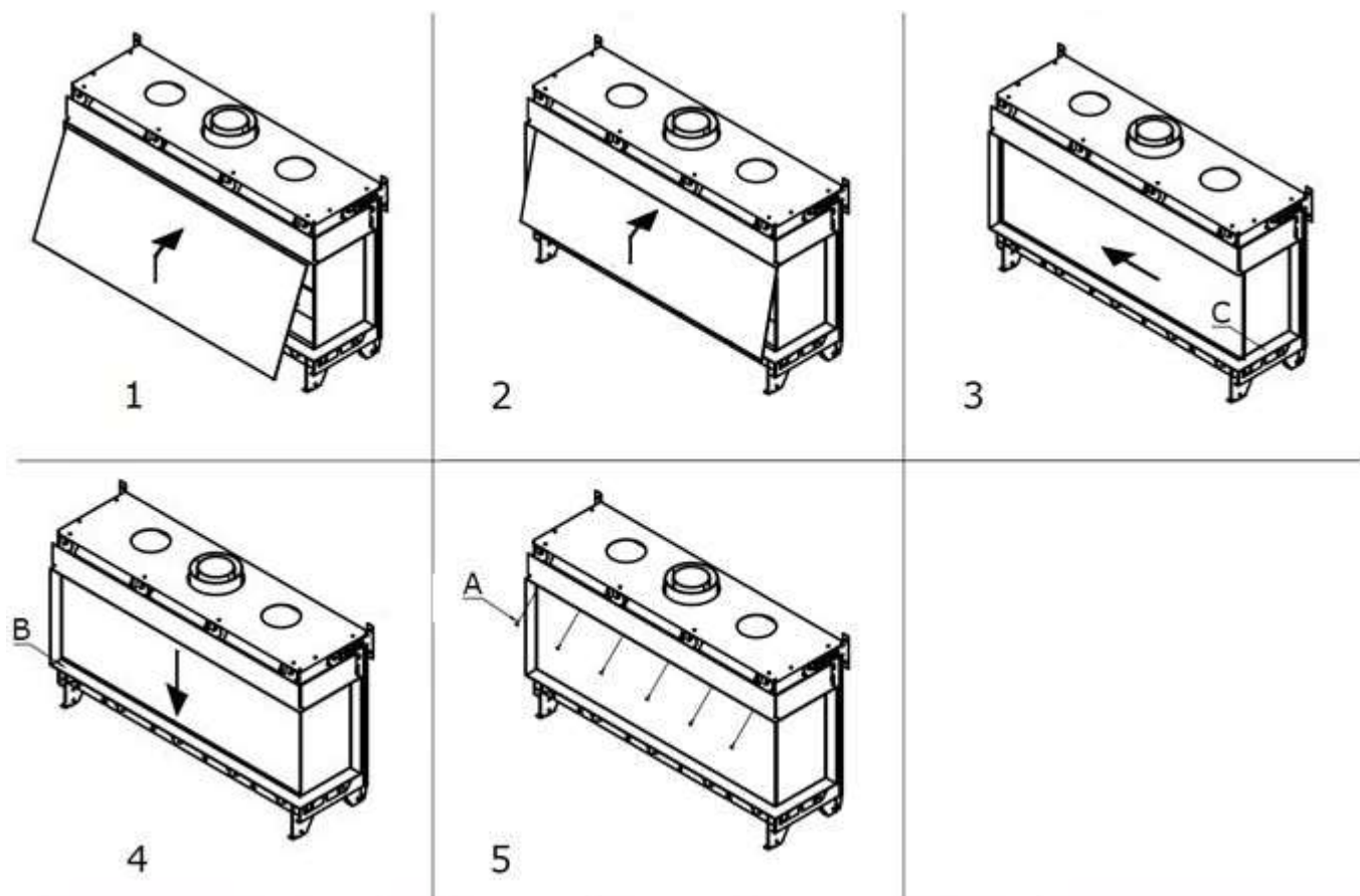
Rysunek 15 – Montaż szyby frontowej w kominku z dwiema szybami
