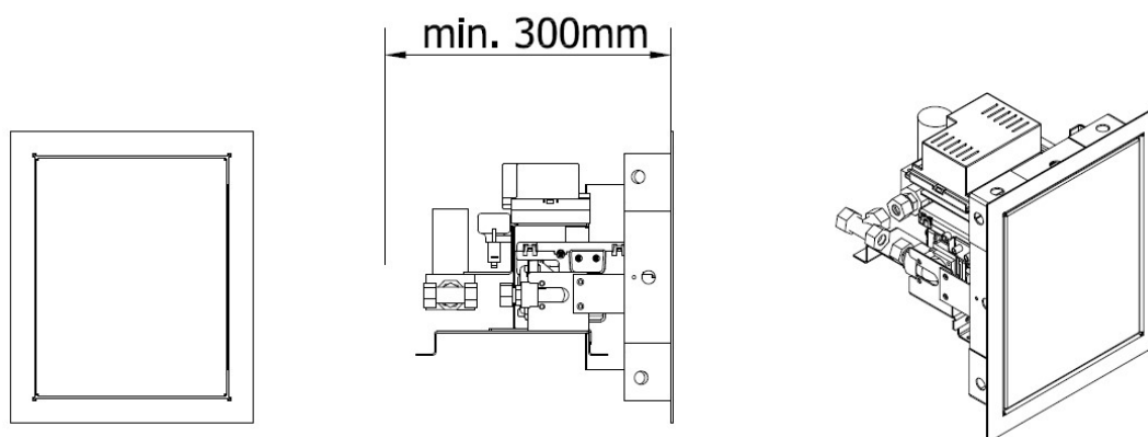
Rysunek 6 – Minimalny wymiar na potrzeby instalacji zespołu gazowego
