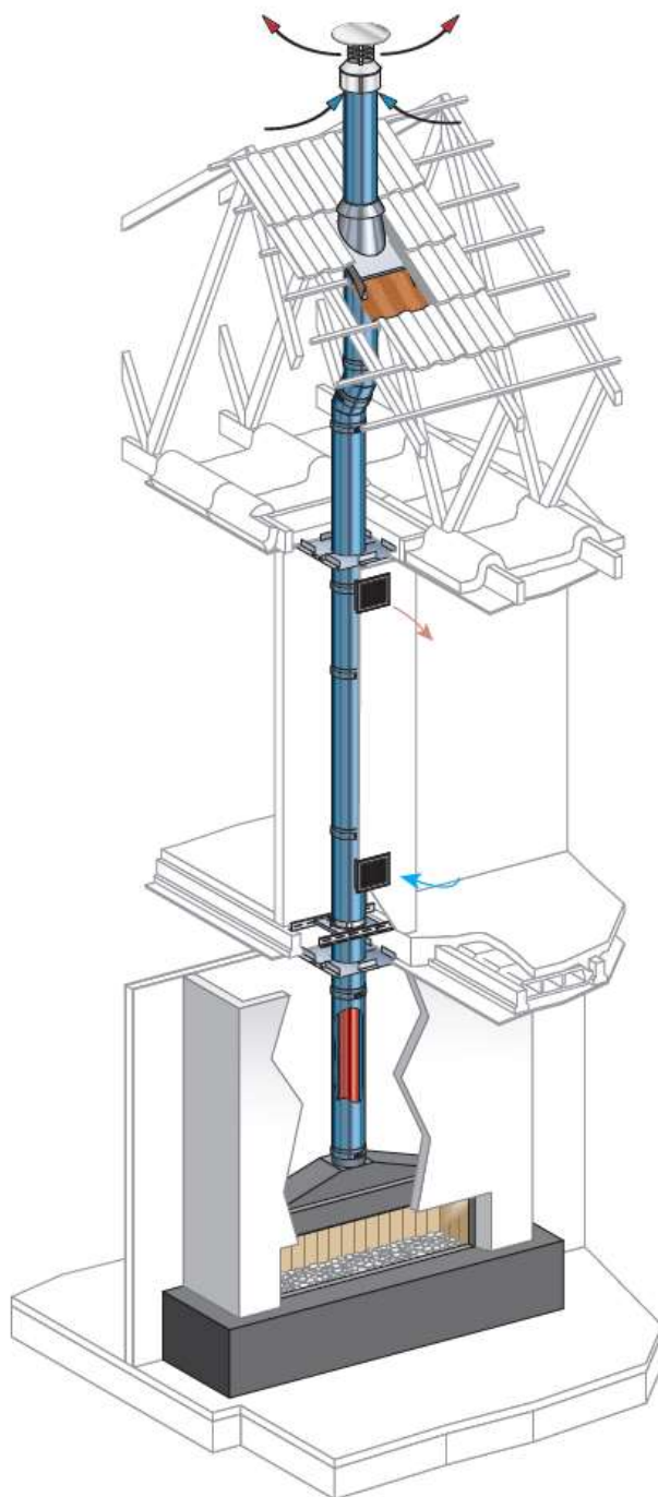
Rysunek 10 – Przykładowa konfiguracja systemu z terminalem dachowym
