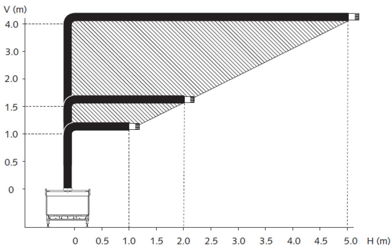
Rysunek 8 - Konfiguracja systemu z terminalem ściennym
