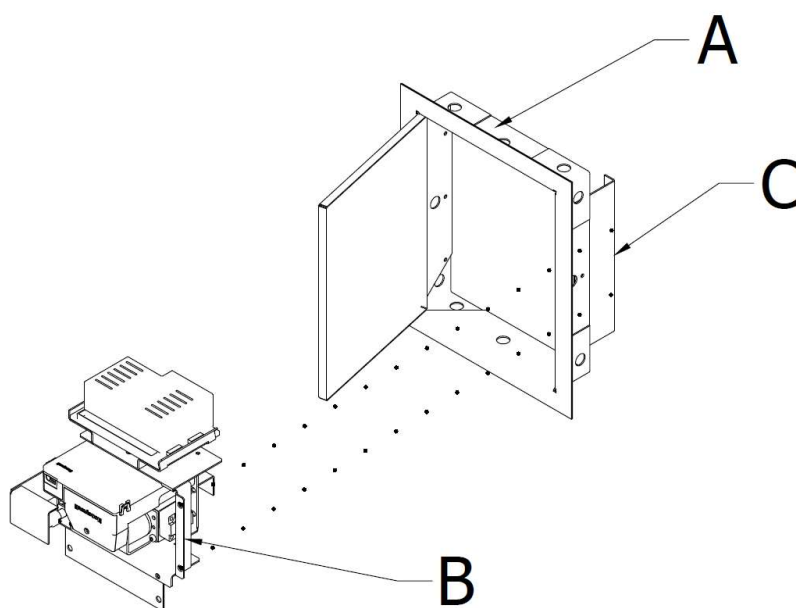
Rysunek 5 - Montaż zespołu gazowego w luku inspekcyjnym
