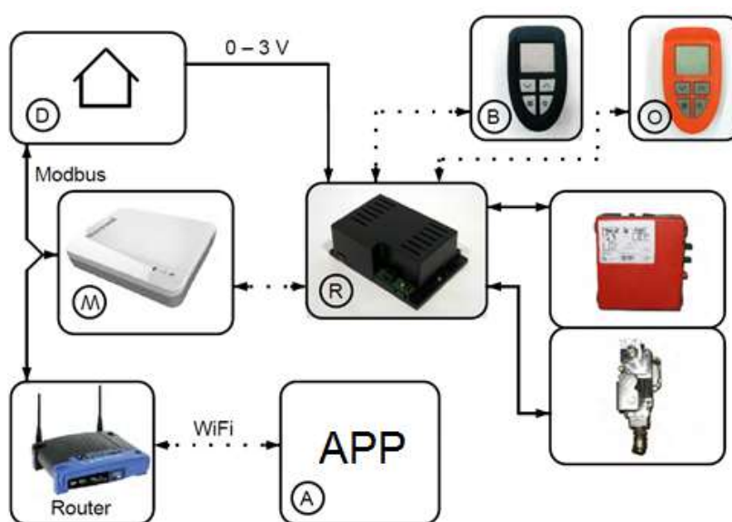
Rysunek 20 – Schemat ideowy elektroniki sterującej
